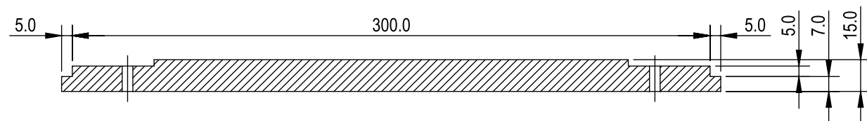
SECTION A-A SCALE 2 : 5
