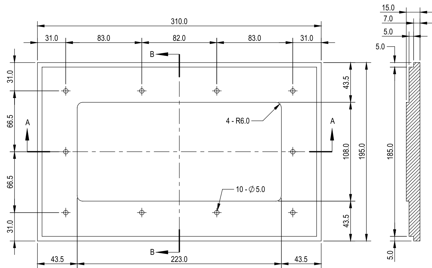
SECTION B-B SCALE 2 : 5
