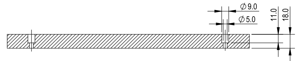
SECTION A-A SCALE 1 : 3
